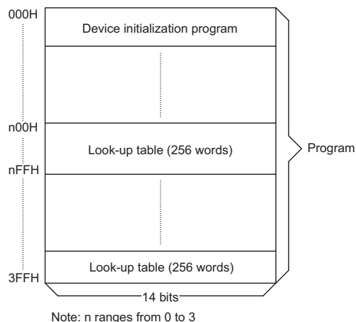
程序存储器
