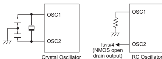
系统振荡器
